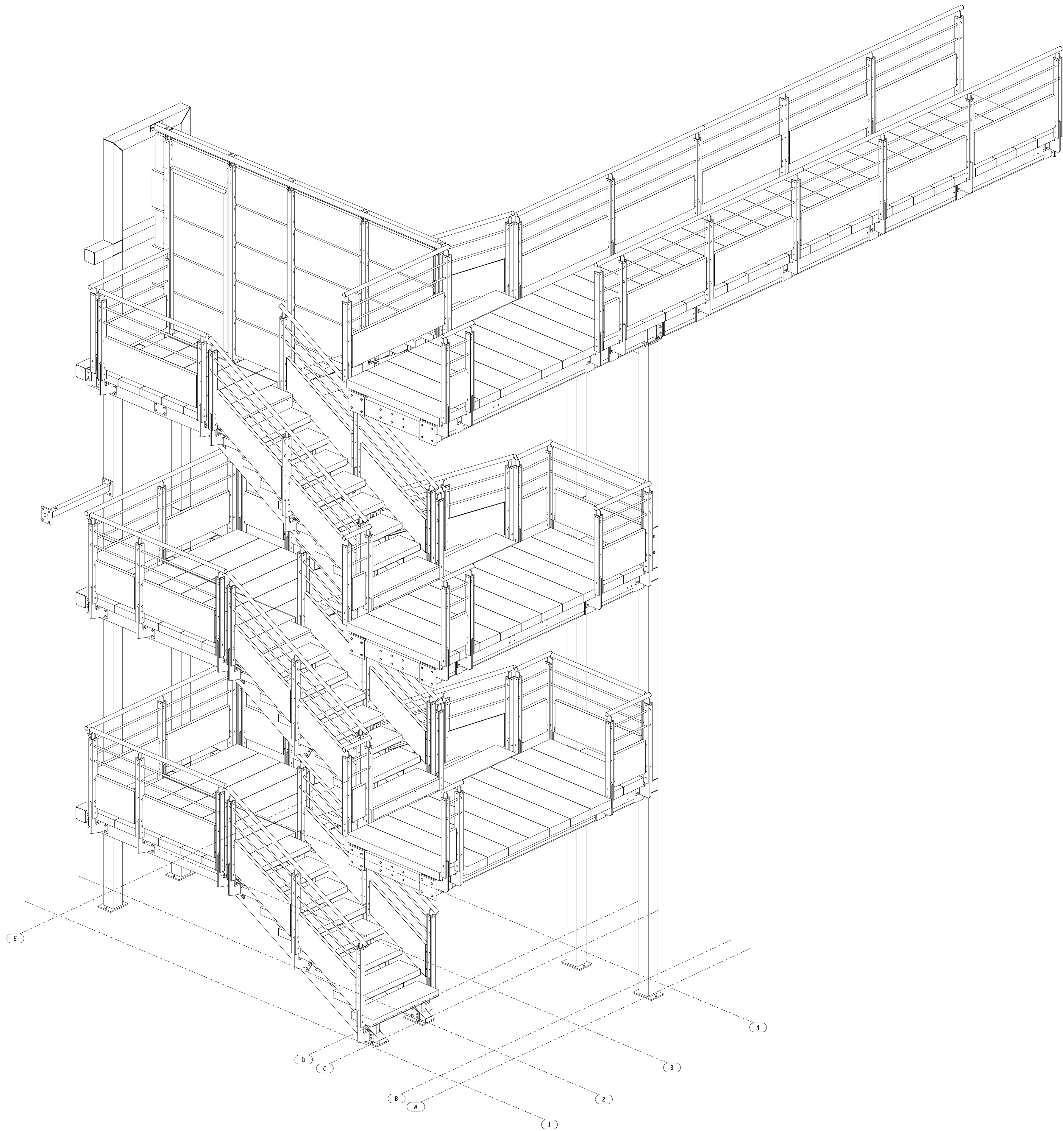
Repérage garde-corps 1:25
