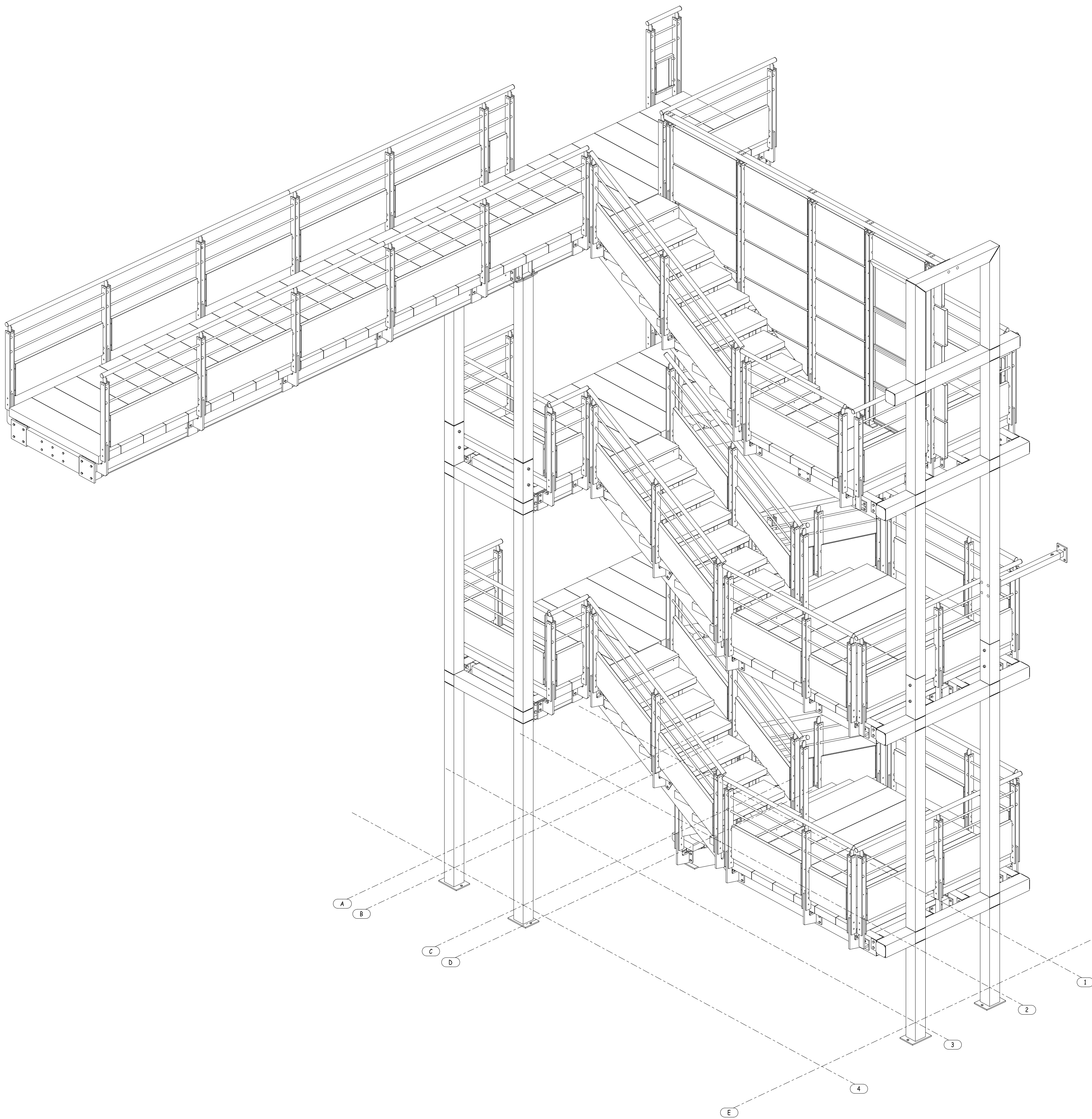
Repérage garde-corps 1:25
